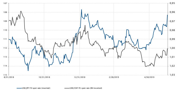
Andamento del tasso di cambio spot USD/JPY e USD/CHF
